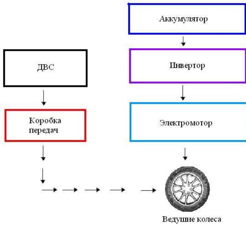
Рисунок 2 Параллельная схема работы гибридного двигателя
